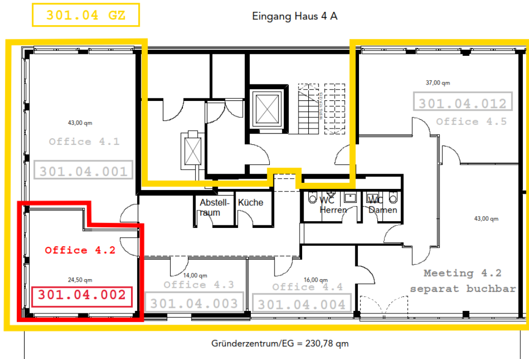
Abbildung 1: Grundriss Mieteinheiten
