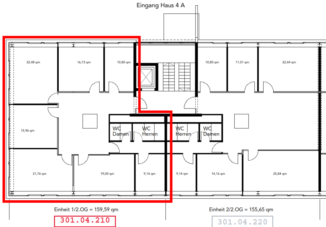
Abbildung 1: Grundriss Mieteinheiten
